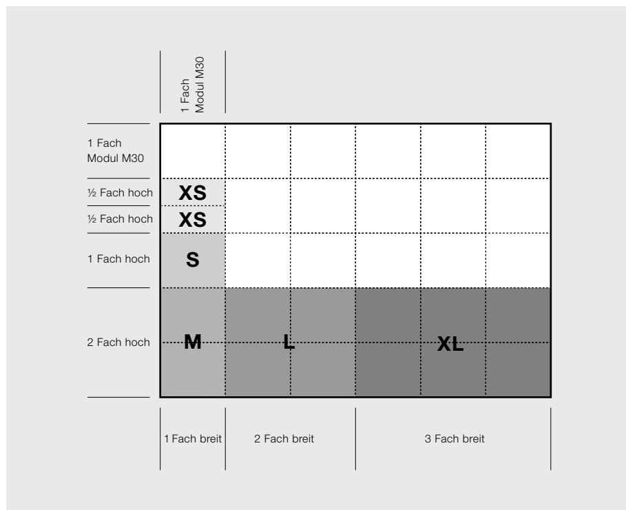
Raster für Zusammenstellung von Briefkästen, Paketboxen und Infoterminal.
